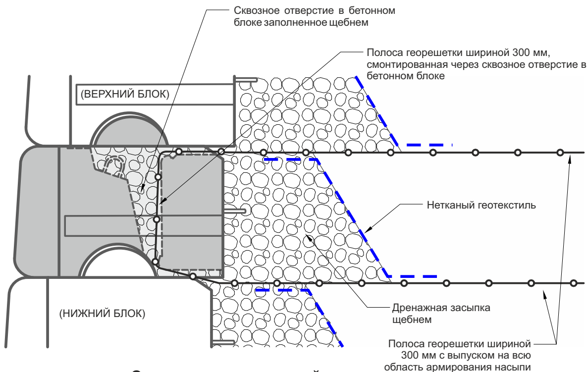
Сечение армогрунтовой конструкции АГ1
